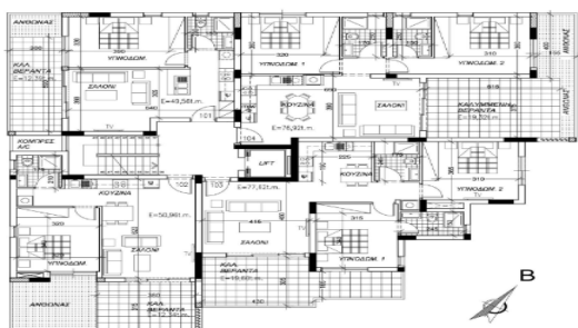
1 ος ΟΡΟΦΟΣ
