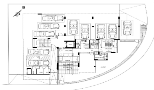
ΙΣΟΓΕΙΟ - ΠΥΛΩΘΗ
