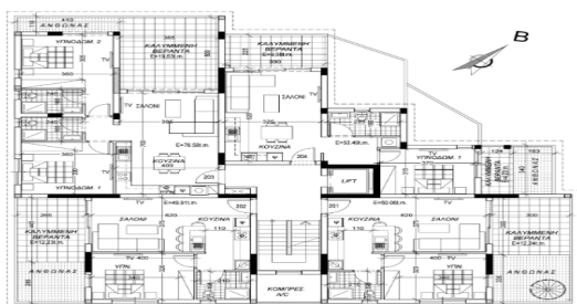
2 ος ΟΡΟΦΟΣ
