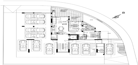
ΙΣΟΓΕΙΟ — ΠΥΛΩΣΗ
