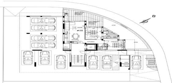
ΑΡΧΙΤΕΚΤΟΝΙΚΑ ΣΧΕΔΙΑ ΙΣΟΓΕΙΟ — ΠΥΛΩΣΗ
