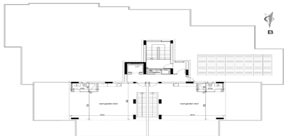
01.000H (ROOF GARDENS)
