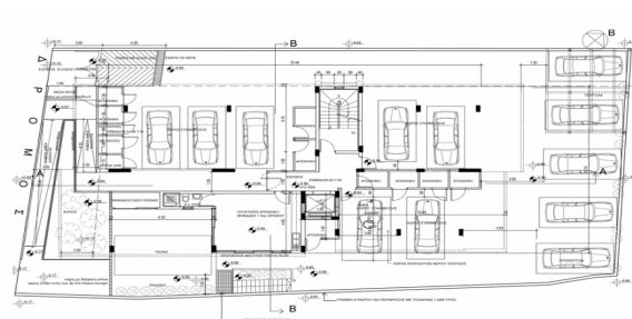
Κατόψη Ισογείου
