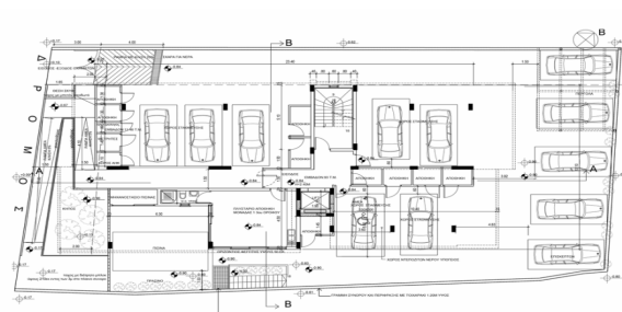
Κατόψη Ισογείου
